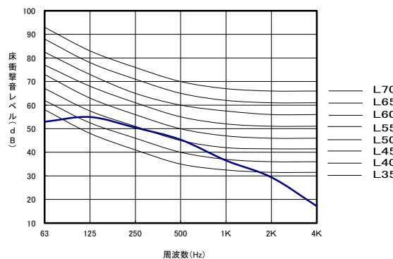
軽量床衝撃音レベル
