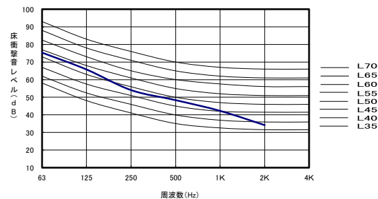
重量床衝撃音レベル
