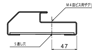
扉枠下部沓摺り枠ビス穴位置
