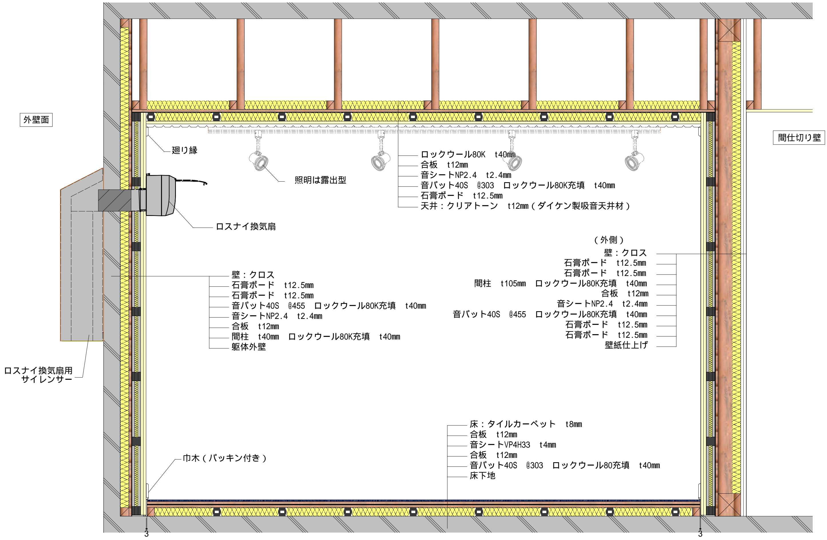
-45dB仕様 断面図 (屋外：-45dB, 間仕切り：-40dB, 上階：-40dB)
