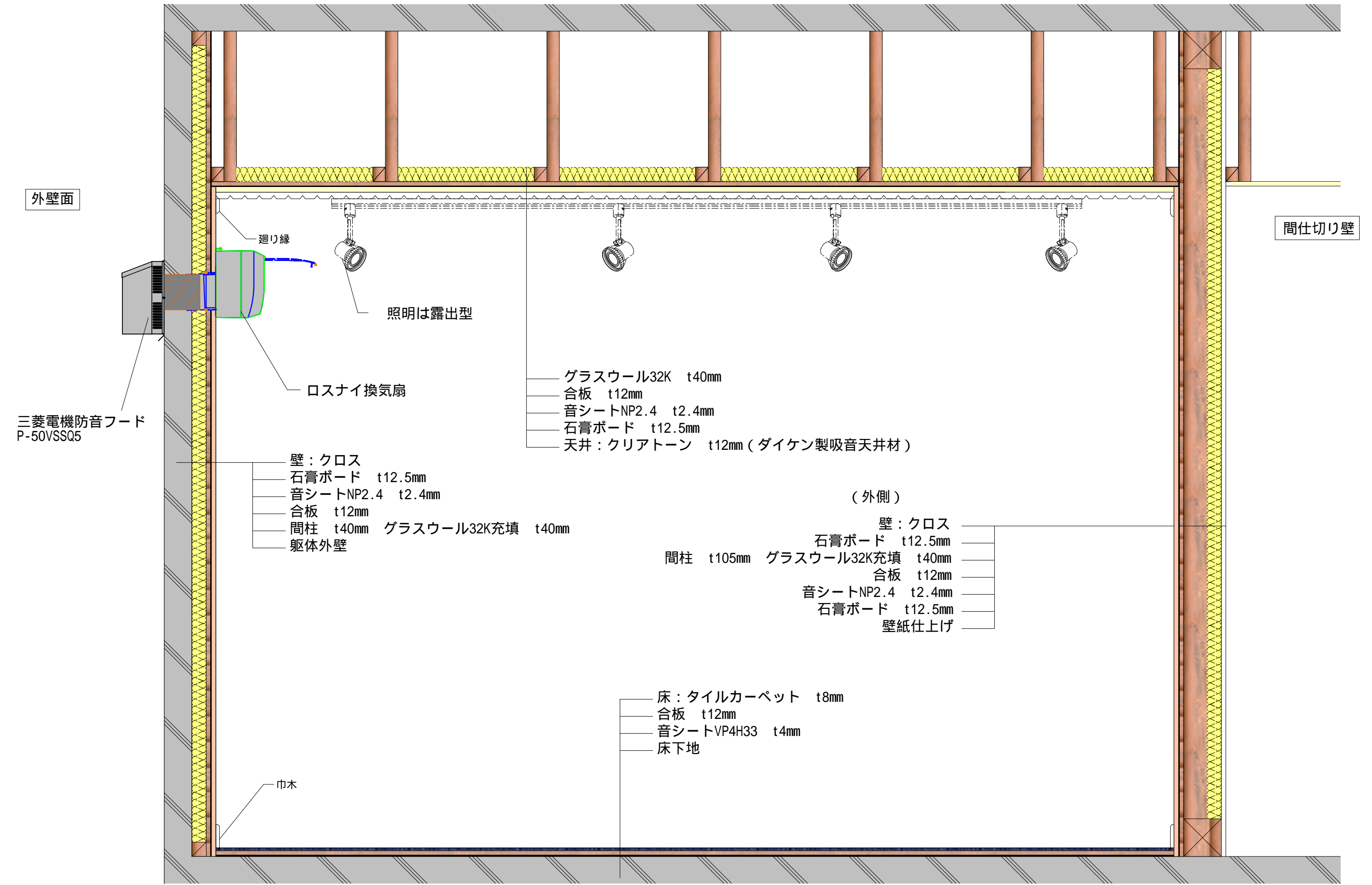
-35dB仕様 断面図 (屋外：-35dB，間仕切り：-35dB，上階：-35dB)
